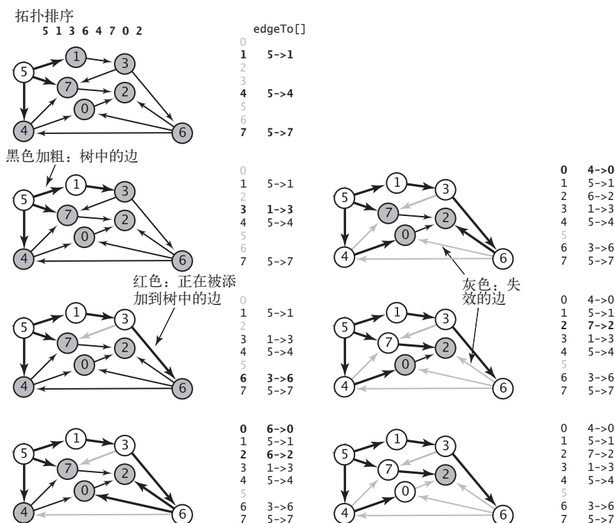
图 4.4.13 寻找无环加权有向图中的最短路径的算法轨迹（另见彩插）
