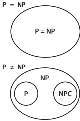
图 6.0.30 问题集的可能情况
