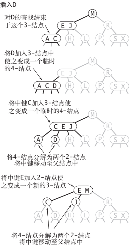
图 3.3.6 向一个父结点为 3-结点的 3-结点中插入新键
