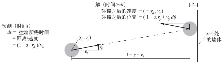
图 6.0.3 预测并解决粒子和墙体的一次碰撞
