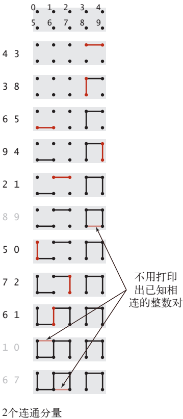
图 1.5.1 动态连通性问题（另见彩插）
