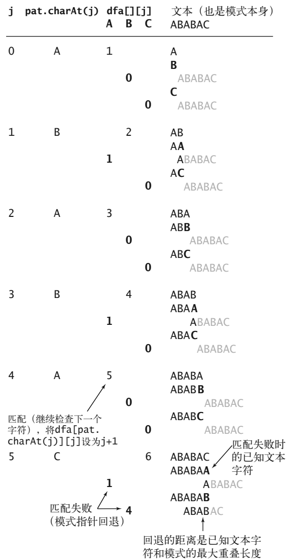
图 5.3.5 KMP 子字符串查找算法在处理 A B A B A C 时模式指针的回退
