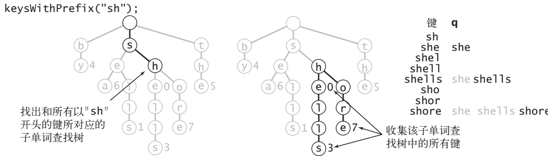
图 5.2.6 单词查找树中的前缀匹配
