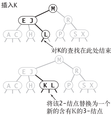
图 3.3.3 向 2- 结点中插入新的键
