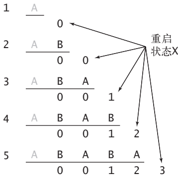
图 5.3.8 计算模式 A B A B A C 的重启状态的 DFA 模拟
