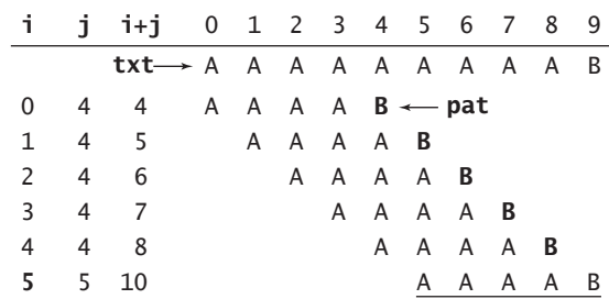
图 5.3.3 暴力子字符串查找（最坏情况）
