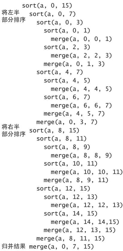
图 2.2.2 自顶向下的归并排序的调用轨迹
