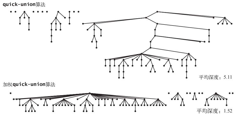
图 1.5.9 quick-union 算法与加权 quick-union 算法的对比（100 个触点，88 次 union() 操作）
