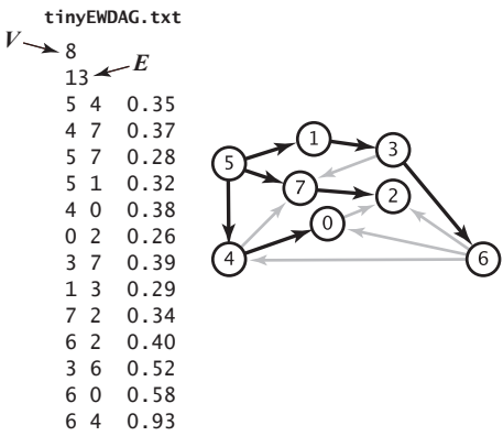
图 4.4.12 一幅无环加权有向图和它的一棵最短路径树
