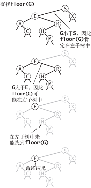
图 3.2.10 计算 floor() 函数
