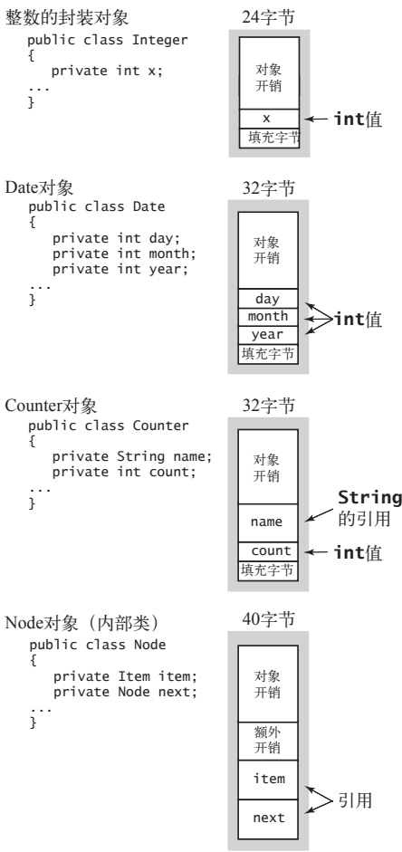
图 1.4.8 典型对象的内存需求
