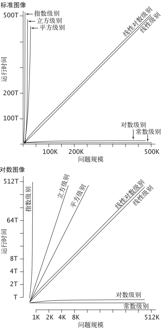
图 1.4.5 典型的增长数量级函数
