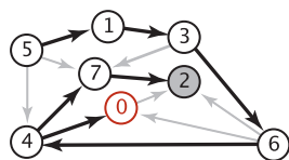
图 4.4.14 无环图中的最长路径算法
