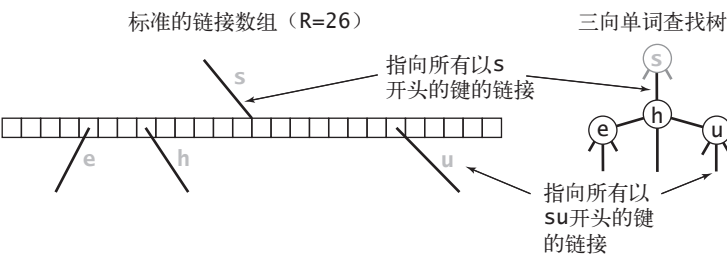
图 5.2.12 单词查找树结点示例
