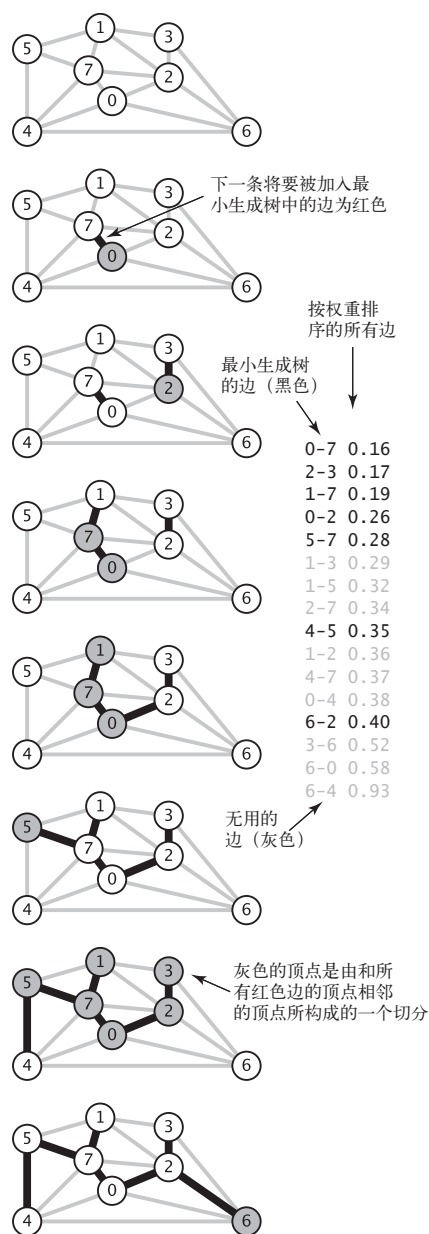
图 4.3.14 Kruskal 算法的轨迹 (另见彩插)
