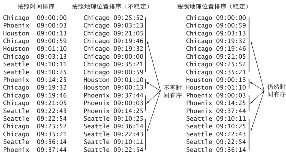
341 图 2.5.1 从另一个键上排序的稳定性
