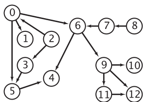
图 4.2.7 标准有向图模型
