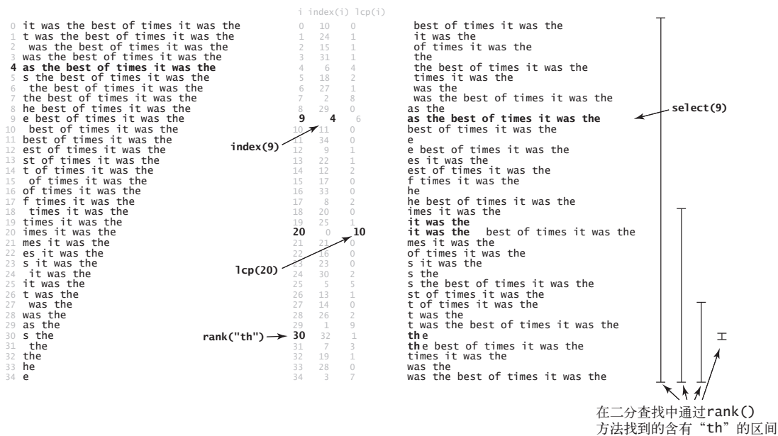
图 6.0.15 后缀数组中的二分查找
