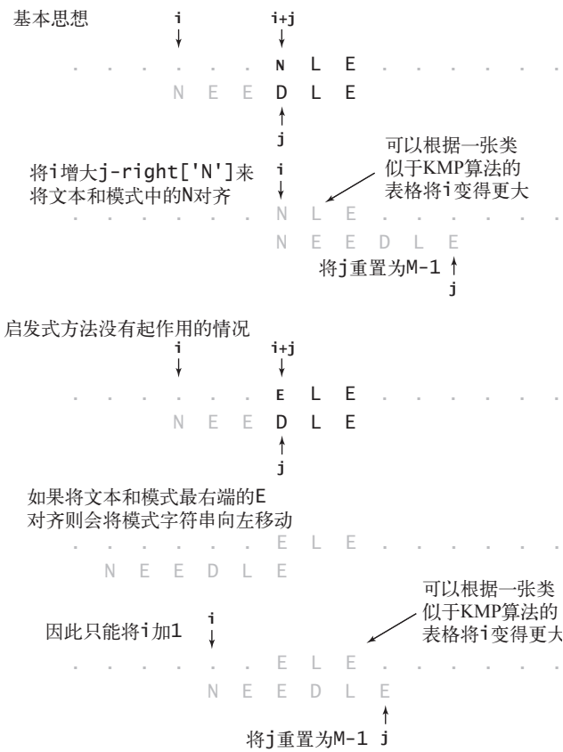
图 5.3.13 启发式的处理不匹配的字符（不匹配的字符包含在模式字符串中）
