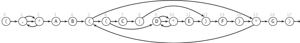
图 5.4.6 模式 (. * AB ((C | D * E) F) * G) 所对应的 NFA
