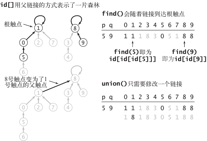
224 图 1.5.4 quick-union 算法概述
