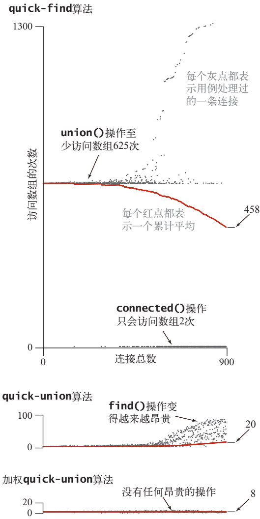
图 1.5.10 所有操作的总成本 (625 个触点, 另见彩插)
