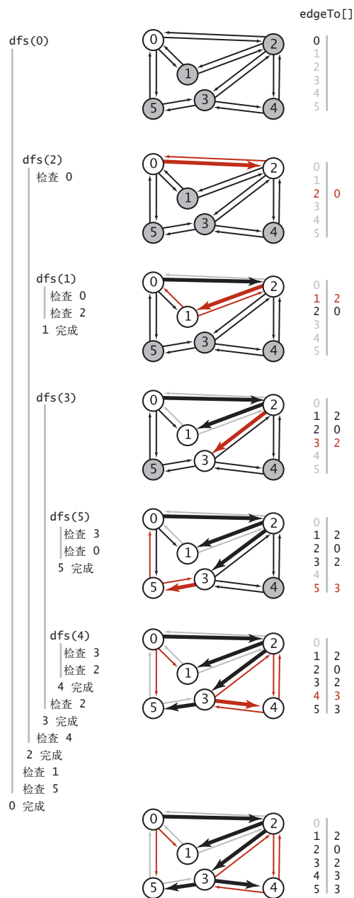
图 4.1.15 使用深度优先搜索的轨迹，寻找所有起点为 0 的路径
