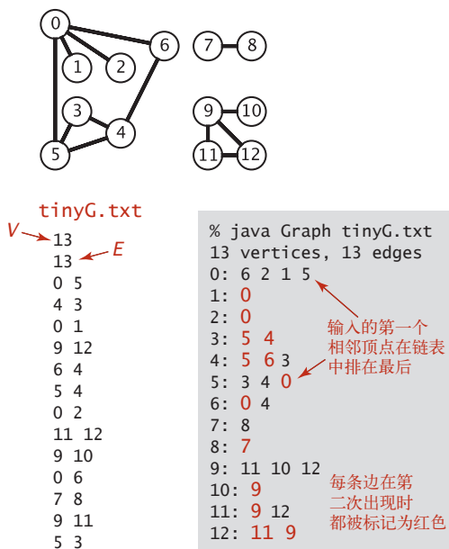
图 4.1.10 由边得到的邻接表
