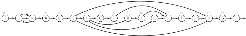
808 图 5.4.8 模式 (.*AB((C|D|E)F)^*G) 所对应的 NFA
