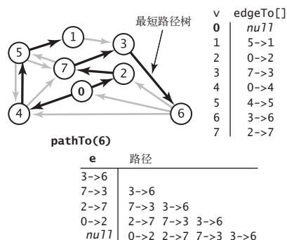
图 4.4.8 pathTo() 方法的计算轨迹
