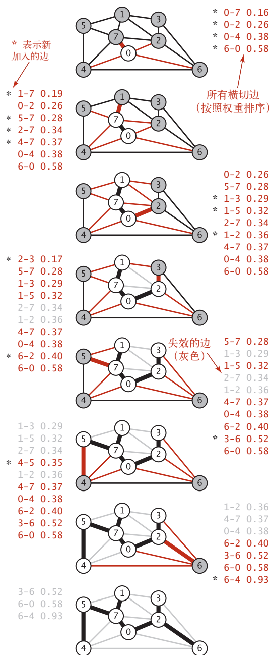
图 4.3.10 Prim 算法的轨迹
