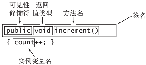
图 1.2.7 详解实例方法
