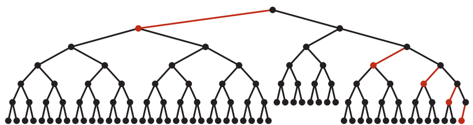
445 图 3.3.28 使用升序键列构造的一棵红黑树，没有画出空链接（另见彩插）
