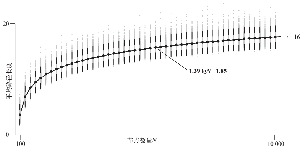
423 图 3.2.14 一棵随机构造的二叉查找树中由根到达任意结点的平均路径长度（另见彩插）
