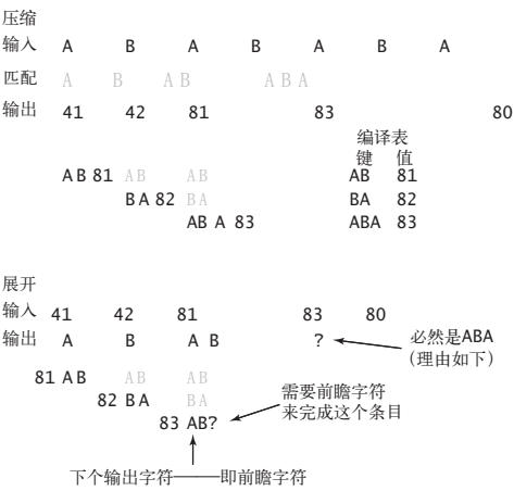
图 5.5.20 LZW 算法的展开：特殊情况
