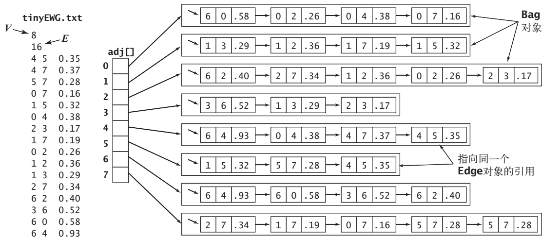
图 4.3.7 加权无向图的表示
