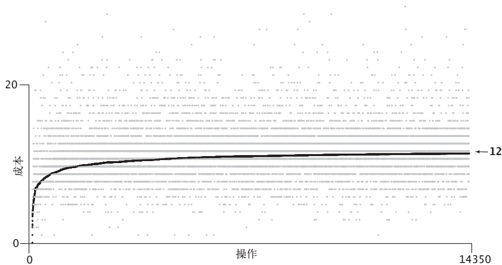
图 3.3.29 使用 RedBlackBST，运行 java FrequencyCounter 8 < tale.txt 的成本
