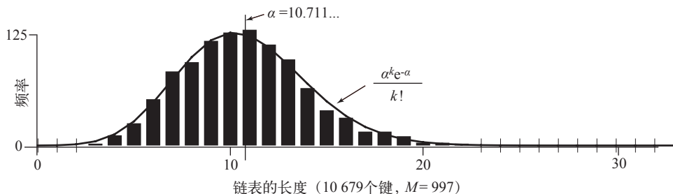
图 3.4.4 使用 SeparateChainingHashST，运行 java FrequencyCounter 8 < tale.txt 时所有链表的长度（另见彩插）
