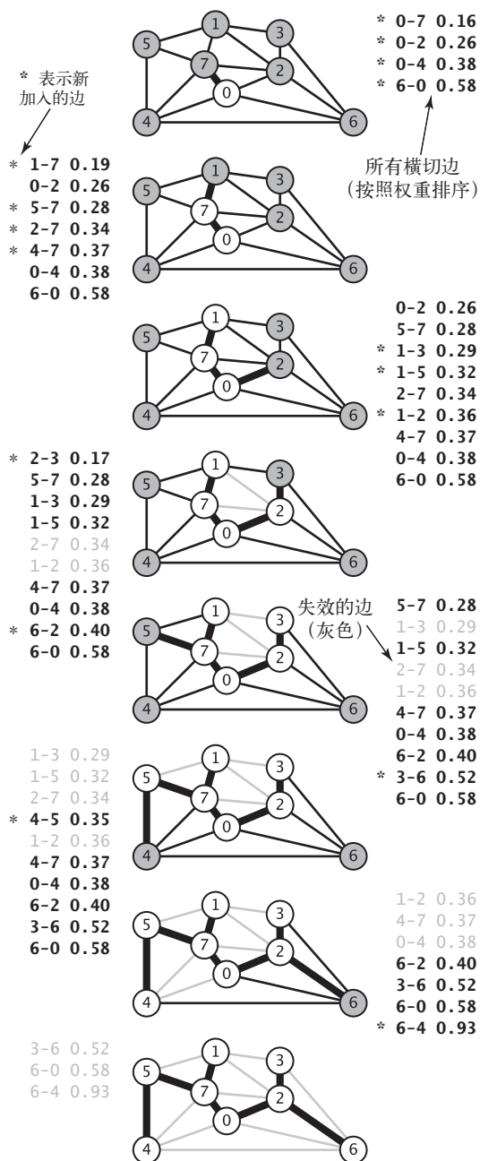
图 4.3.10 Prim 算法的轨迹（延时实现，另见彩插）
