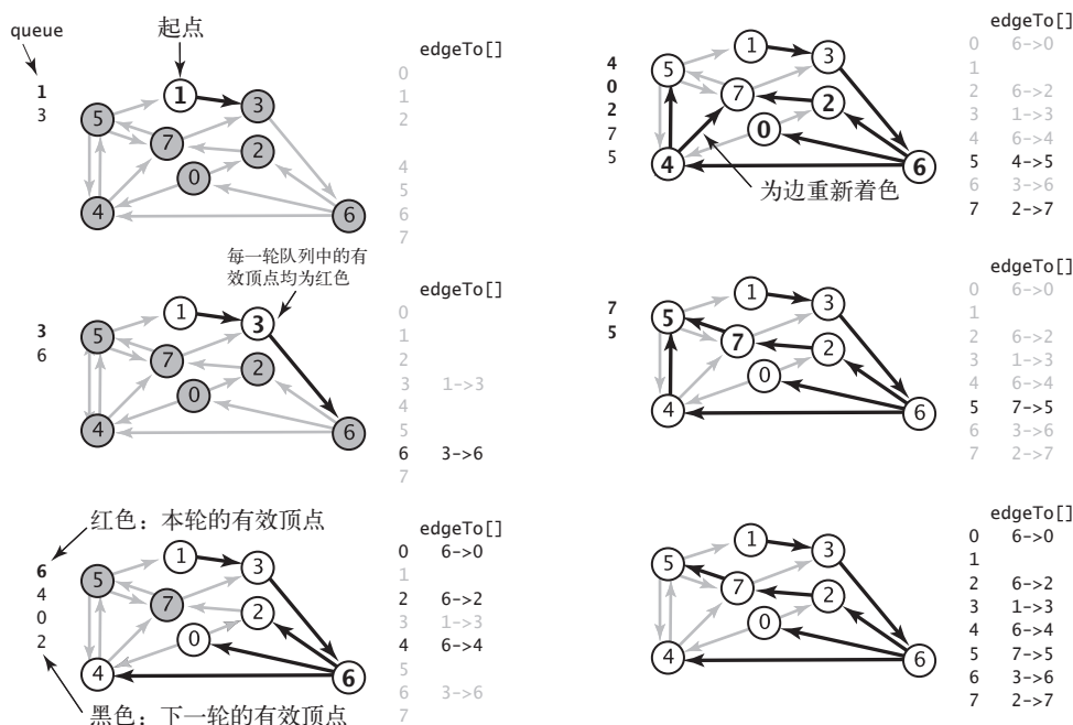
图 4.4.22 Bellman-Ford 算法的轨迹 (另见彩插)
