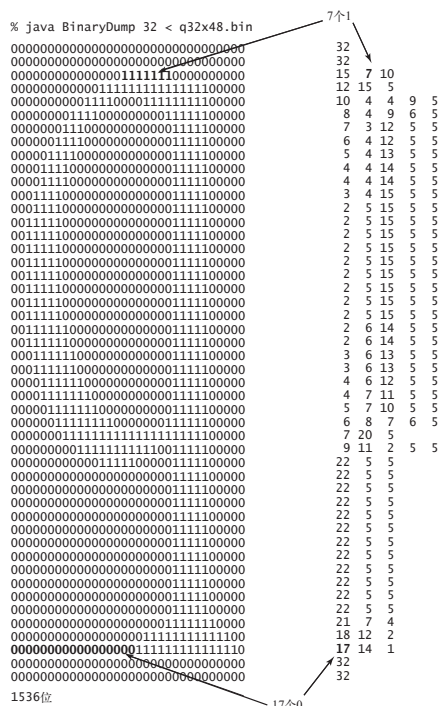
图 5.5.8 一幅典型的位图，每行的游程编码如右所示
