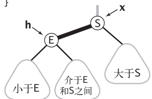
图 3.3.16 左旋转 h 的右链接（另见彩插）
