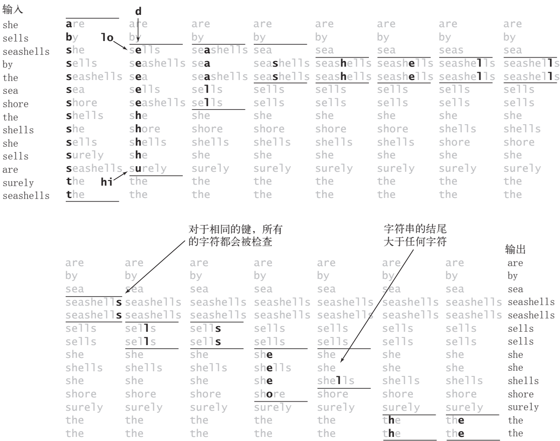
图 5.1.12 高位优先的字符串排序的递归调用轨迹（小数组不会切换到插入排序，大小为 0 和 1 的子数组已被省略）
