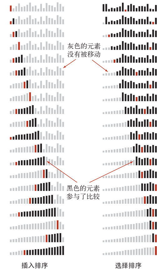
图 2.1.1 初级排序算法的可视轨迹图（另见彩插）
