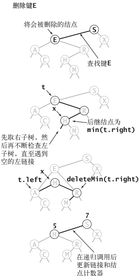
图 3.2.13 二叉查找树中的删除操作
