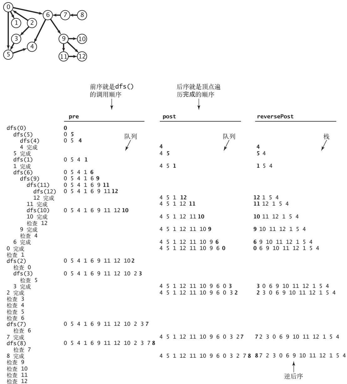
图 4.2.10 计算有向图中顶点的深度优先次序（前序、后序和逆后序）
