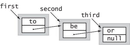
图 1.3.5 用链接构造一条链表
