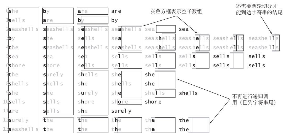
图 5.1.17 三向字符串快速排序的递归调用轨迹（不在子数组较小时切换排序方法）
