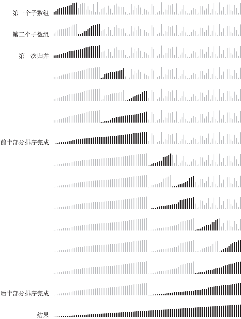
图 2.2.4 改进了小规模子数组排序方法后的自顶向下的归并排序的可视轨迹
