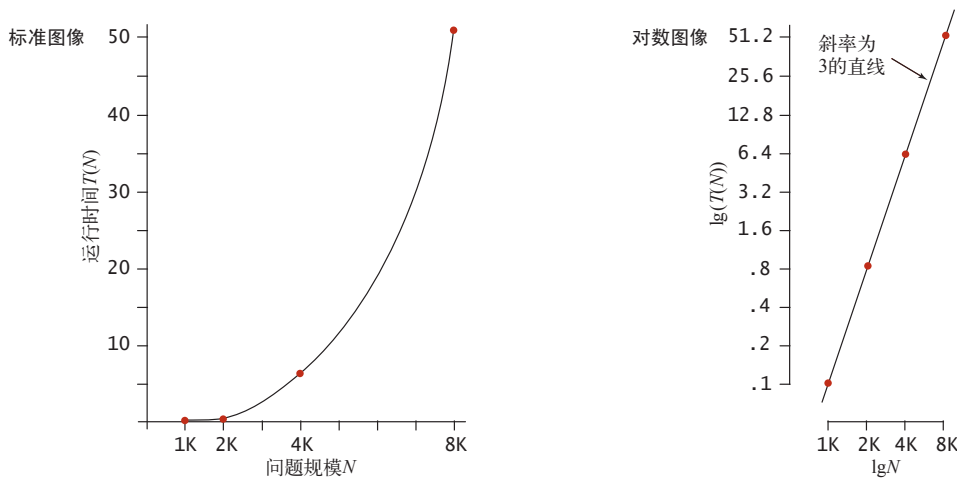
图 1.4.2 实验数据 (ThreeSum.count()) 的运行时间) 的分析
