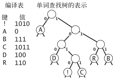
图 5.5.11 一种霍夫曼编码
