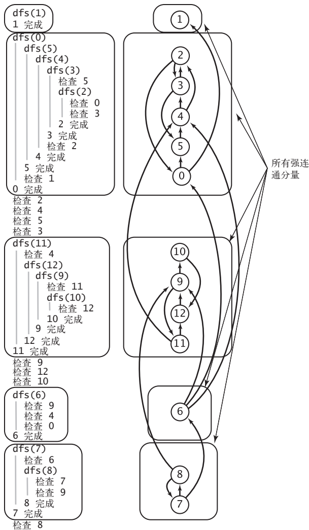
图 4.2.16 在有向图中寻找强连通分量的 Kosaraju 算法
