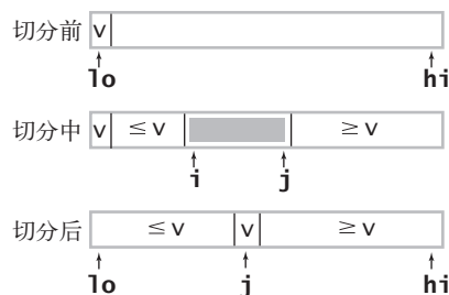
图 2.3.2 快速排序的切分示意图
