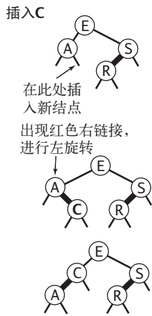
图 3.3.19 向树底部的 2- 结点插入一个新键 (另见彩插)
