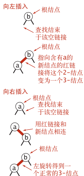
图 3.3.18 向单个 2- 结点中插入一个新键
