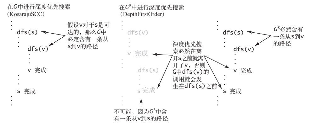
图 4.2.15 Kosaraju 算法的正确性证明
