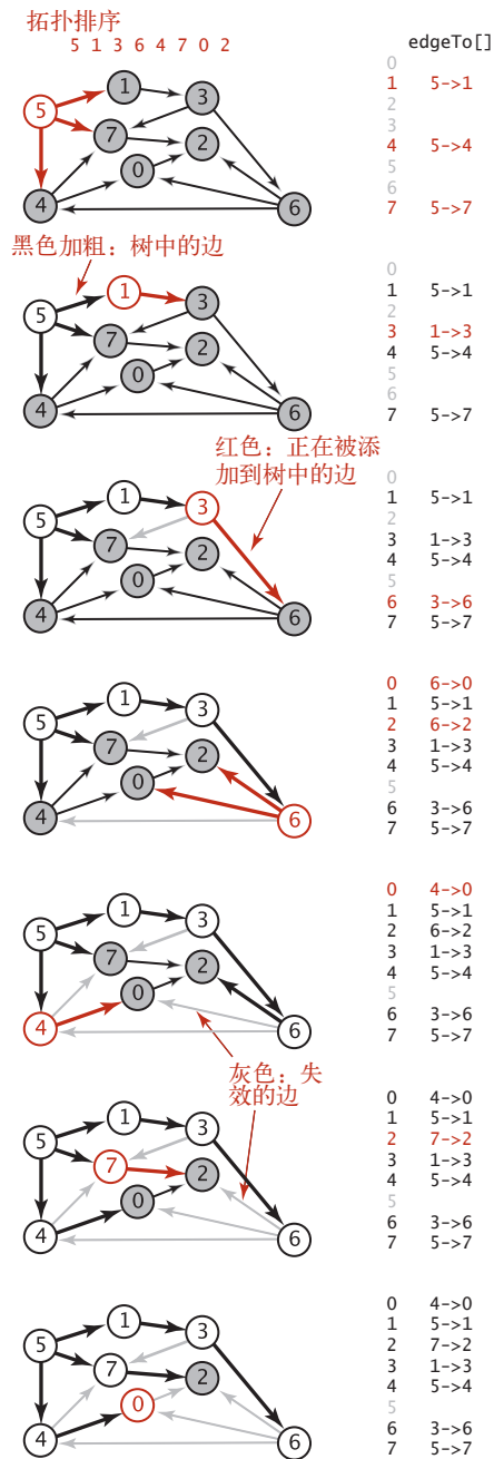
图 4.4.13 寻找无环加权有向图中的最短路径的算法轨迹
