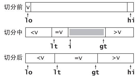
图 2.3.4 三向切分的示意图
