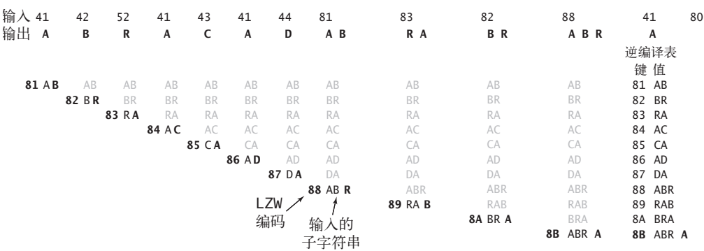
841 图 5.5.19 LZW 算法对 41 42 52 41 43 41 44 81 83 82 88 41 80 的展开
