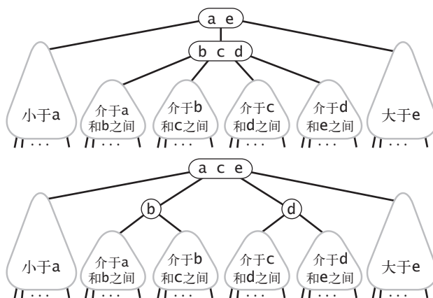
图 3.3.9 4- 结点的分解是一次局部变换，不会影响树的有序性和平衡性
