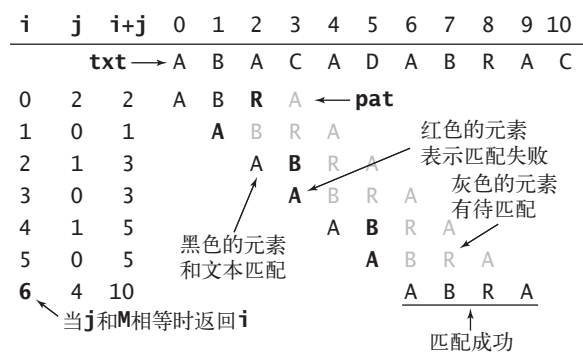
图 5.3.2 暴力子字符串查找（另见彩插）
