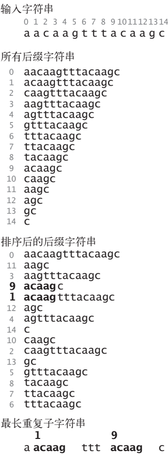
图 6.0.12 使用后缀排序计算最长重复子字符串
