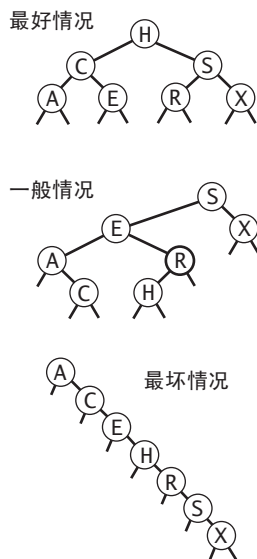
图 3.2.7 二叉查找树的可能形状
