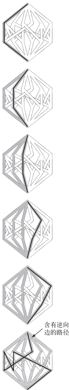
图 6.0.26 二分图匹配中的增广路径
