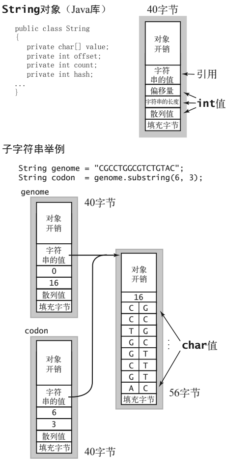
图 1.4.10 一个 String 对象和一个子字符串
