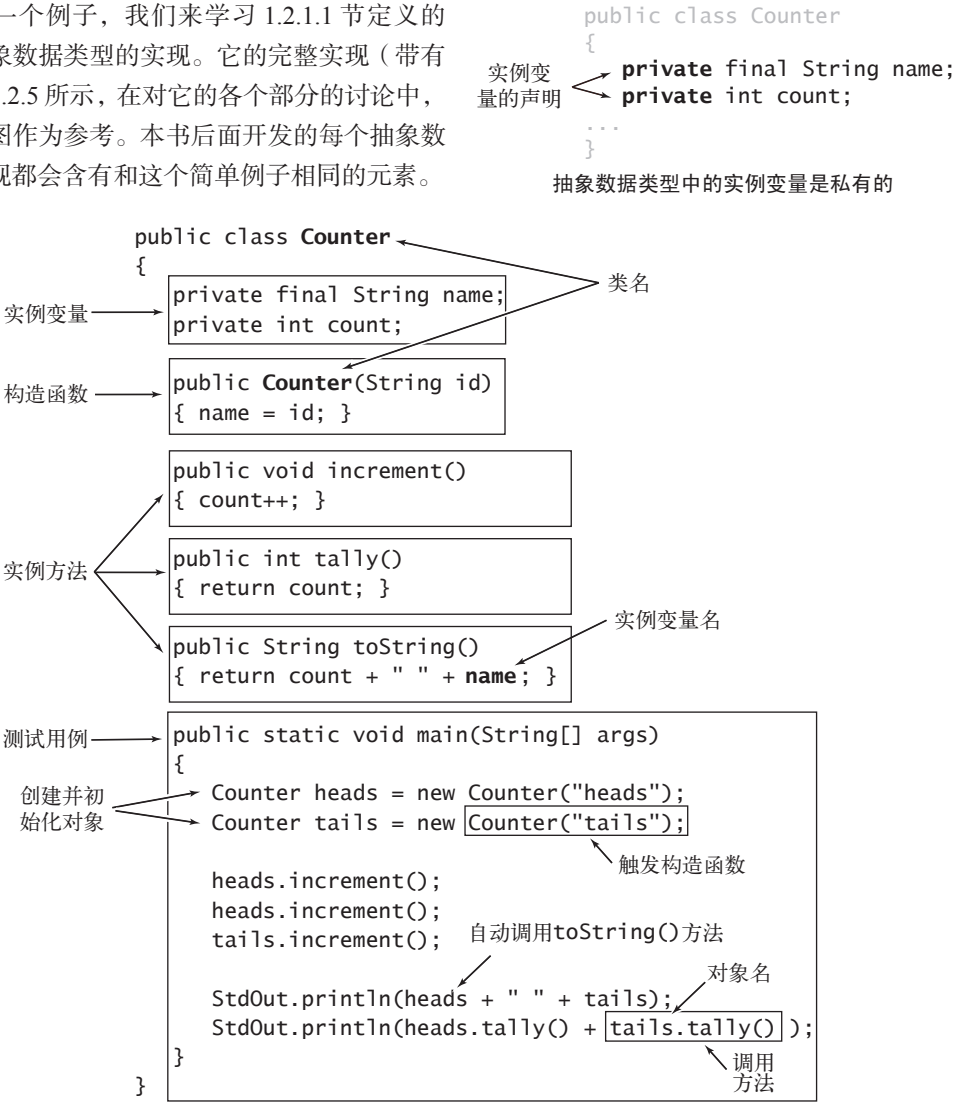
图 1.2.5 详解数据类型的定义类
