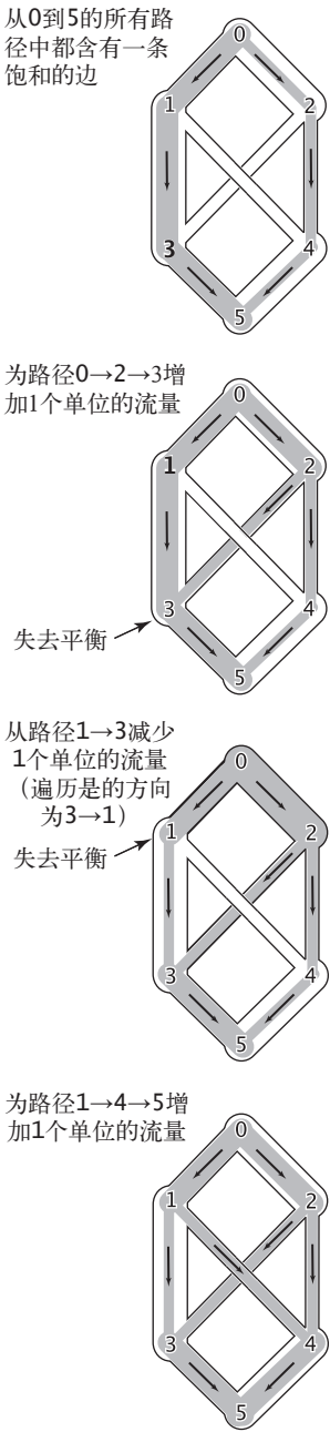
图 6.0.21 一条增广路径 (0 → 2 → 3 → 1 → 4 → 5)
