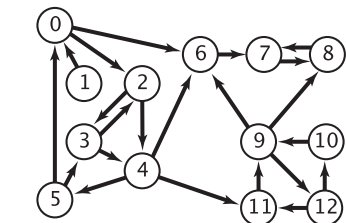
在反向图中进行深度优先搜索(ReversePost)
