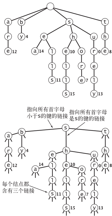
图 5.2.10 一棵单词查找树所对应的三向单词查找树
