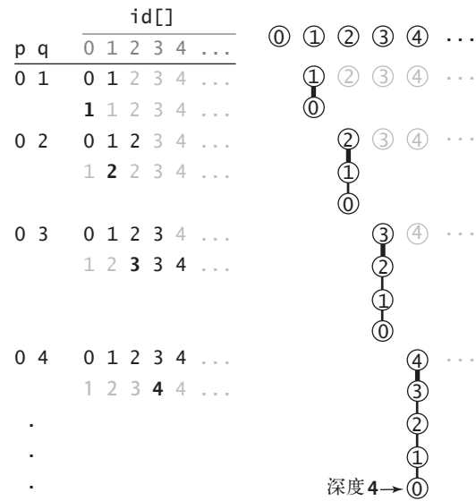
图 1.5.6 quick-union 算法的最坏情况
