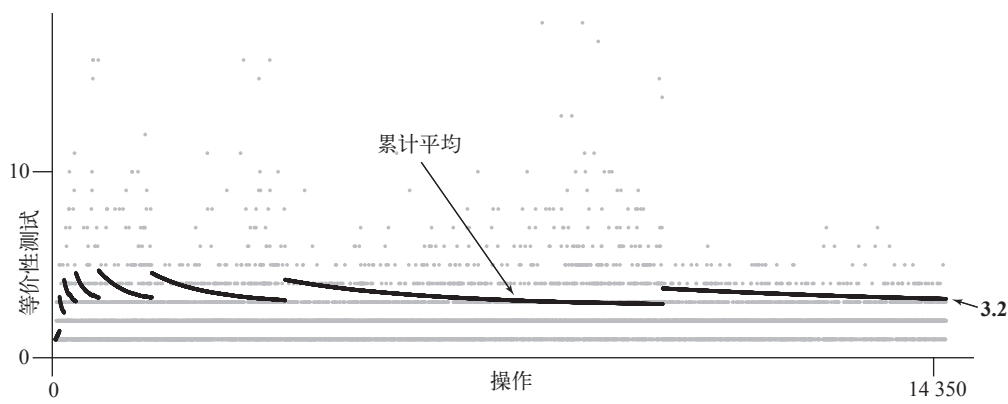
475 图 3.4.10 使用能够自动调整数组大小的 LinearProbingHashST，运行 java FrequencyCounter 8 < tale.txt 的成本
