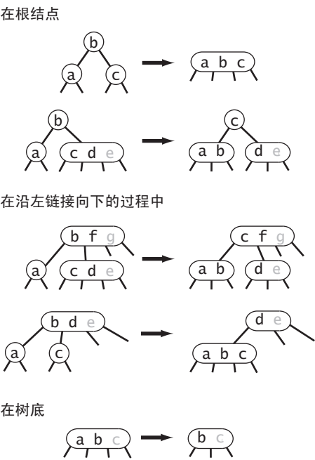
图 3.3.26 删除最小键操作中的变换
