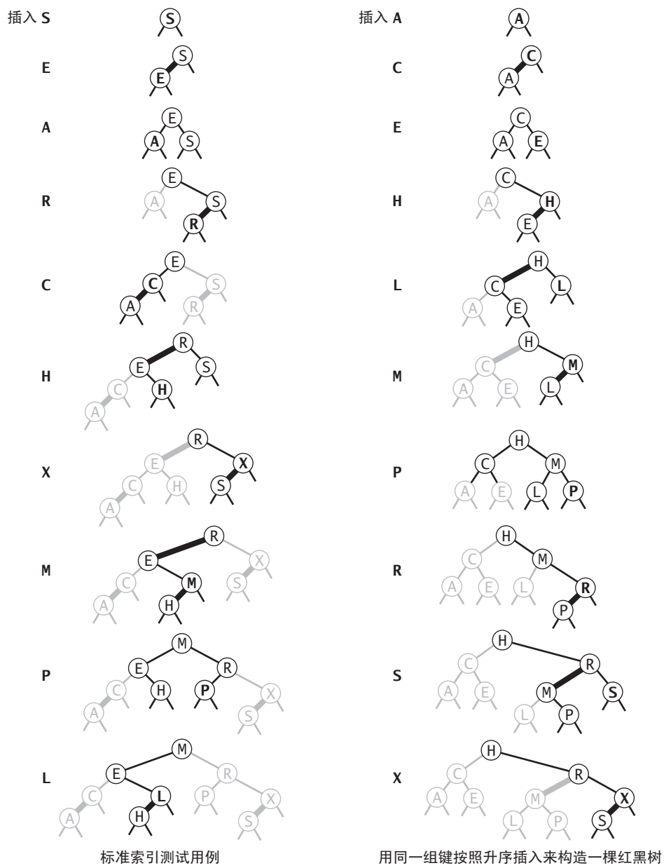
图 3.3.24 红黑树的构造轨迹（另见彩插）
