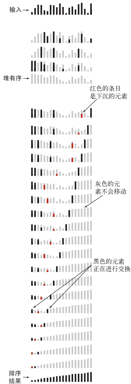
图 2.4.8 堆排序的可视轨迹 (另见彩插)
