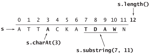
图 5.0.1 String 类型的基本常数时间操作
