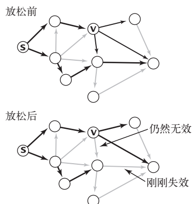
图 4.4.7 顶点的松弛
