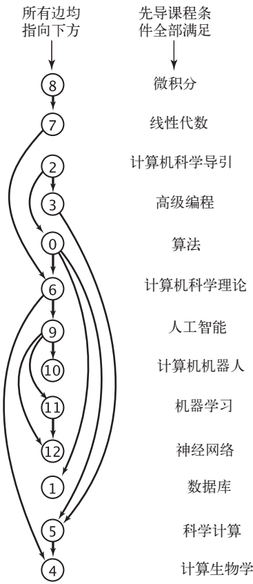
图 4.2.8 拓扑排序
