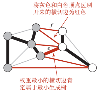
图 4.3.4 切分定理
