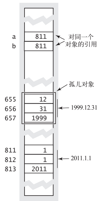
图 1.2.9 孤儿对象
