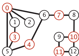
图 4.1.7 二分图
