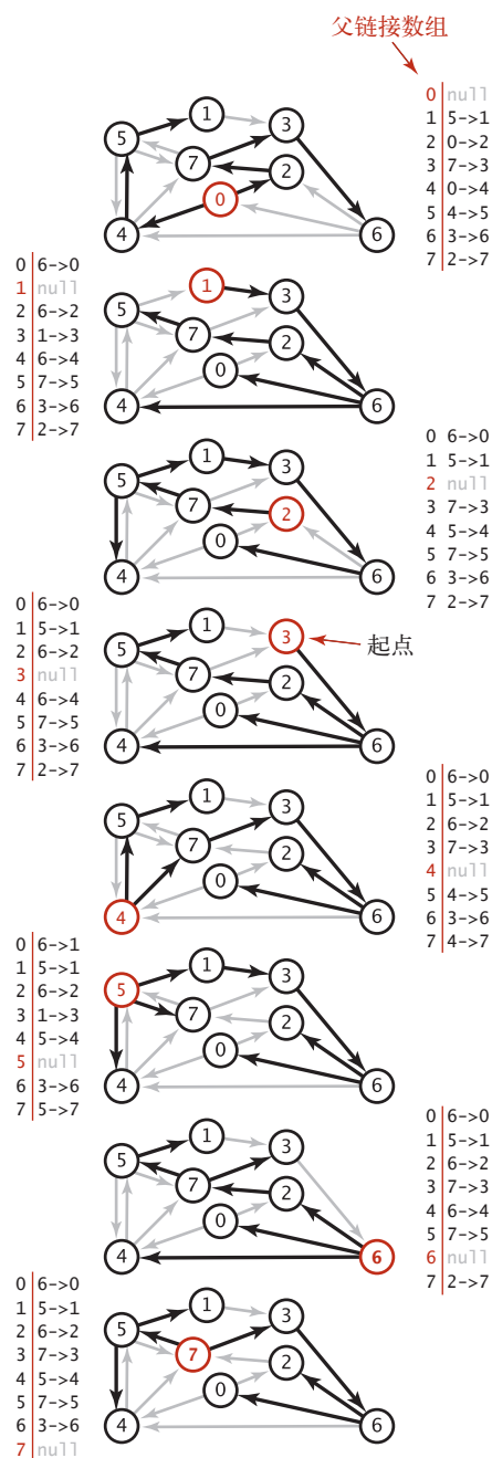
图 4.4.2 最短路径树
