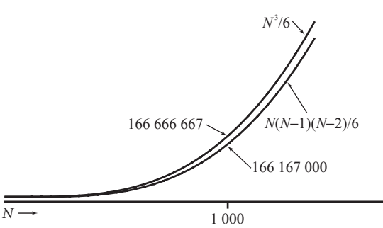
图 1.4.3 首项近似
