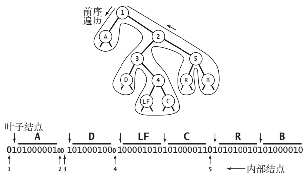
图 5.5.14 使用前序遍历将一棵单词查找树编码为比特流
