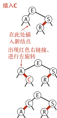
图 3.3.19 向树底部的 2- 结点插入一个新键
