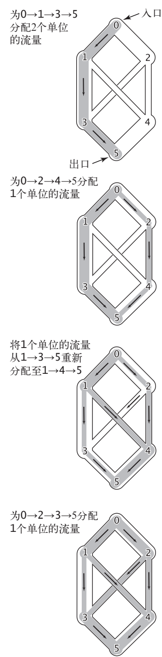
图 6.0.17 为输油网络分配流量
