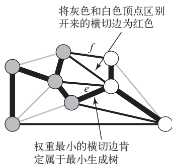
图 4.3.4 切分定理（另见彩插）
