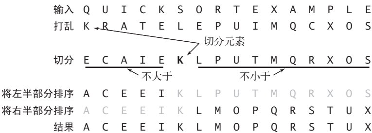
288 图 2.3.1 快速排序示意图
