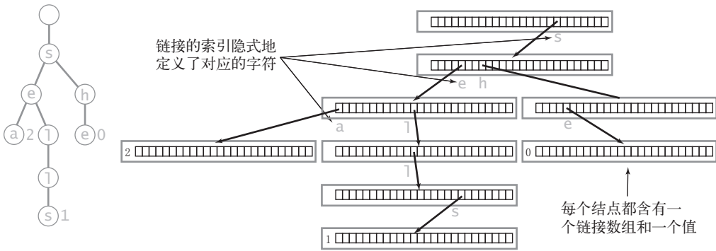
图 5.2.4 单词查找树的表示 ( R=26 )
