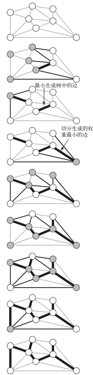
图 4.3.6 贪心最小生成树算法 (另见彩插)
