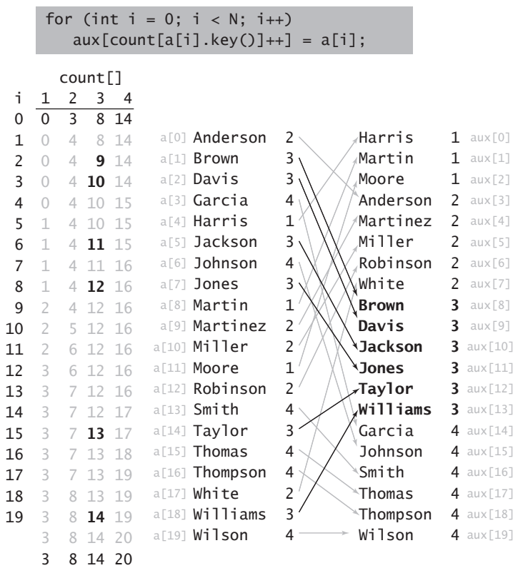
图 5.1.4 将数据分类（键为 3 的条目均突出显示）
