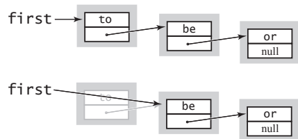
图 1.3.7 删除链表的首结点
