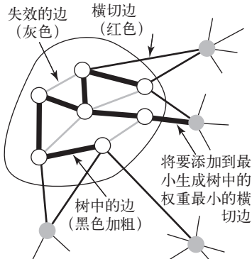
图 4.3.9 最小生成树的 Prim 算法（另见彩插）
