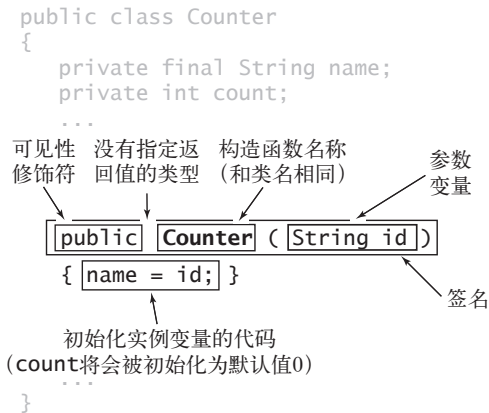
图 1.2.6 详解构造函数
