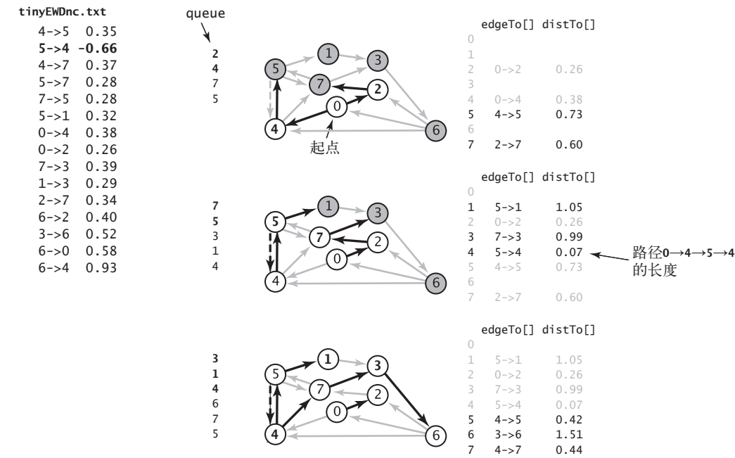
图 4.4.25 Bellman-Ford 算法的轨迹（含有负权重环的图，另见彩插）
