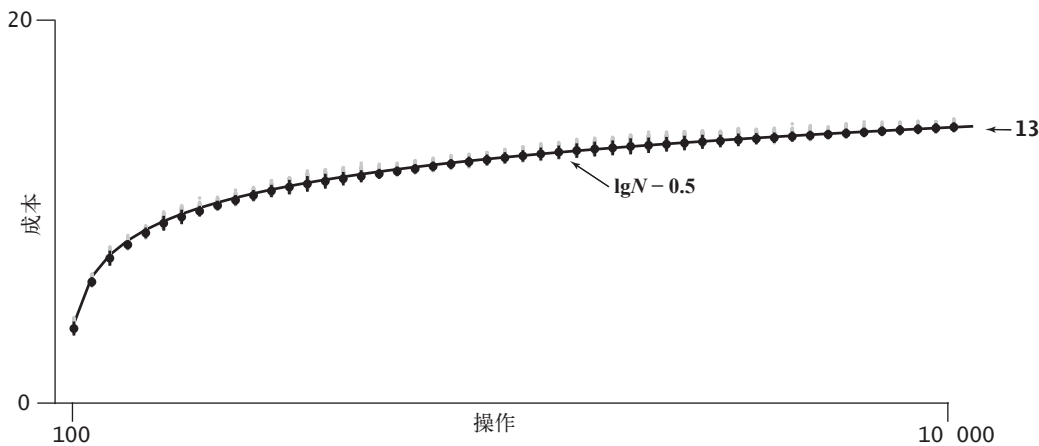
456 图 3.3.30 随机构造的红黑树中到达一个随机结点的平均路径长度（另见彩插）
