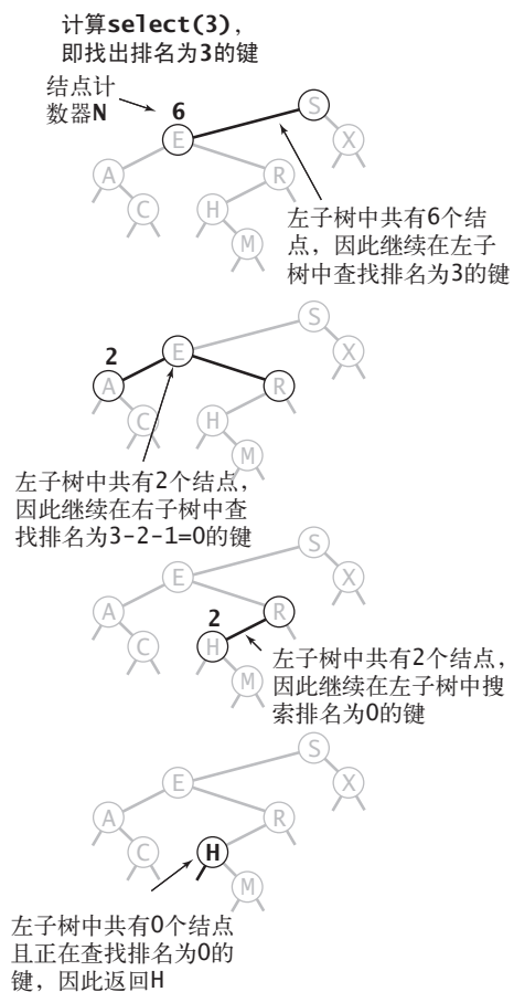
图 3.2.11 二叉查找树中的 select() 操作
