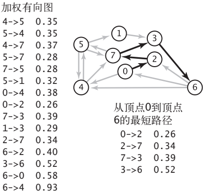
图 4.4.1 一幅加权有向图和其中的一条最短路径
