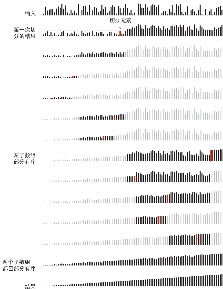
297 图 2.3.3 使用了三取样切分和插入排序转换的快速排序（另见彩插）
