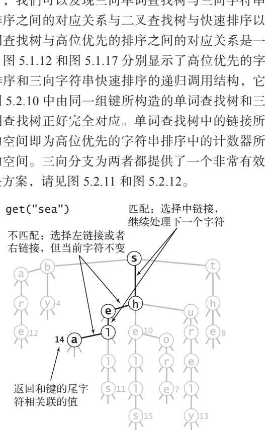
图 5.2.11 三向单词查找树中的查找示例
