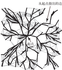
图 4.4.3 一棵含有 250 个顶点的最短路径树
