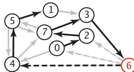
图 4.4.24 Bellman-Ford 算法的轨迹 (图中含有负权重边)
