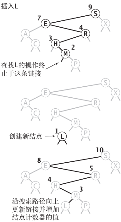
图 3.2.5 二叉查找树的插入操作
