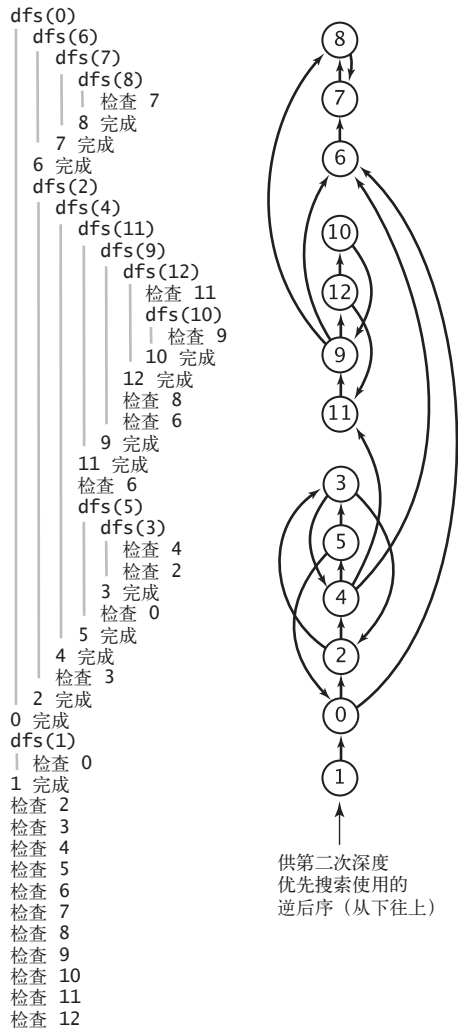
图 4.2.16 在有向图中寻找强连通分量的 Kosaraju 算法
