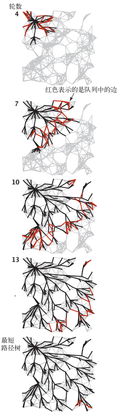
图 4.4.23 Bellman-Ford 算法（250 个顶点）（另见彩插）
