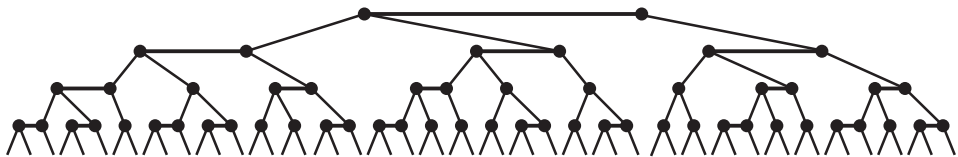
432 图 3.3.13 将红链接画平时，一棵红黑树就是一棵 2-3 树（另见彩插）
