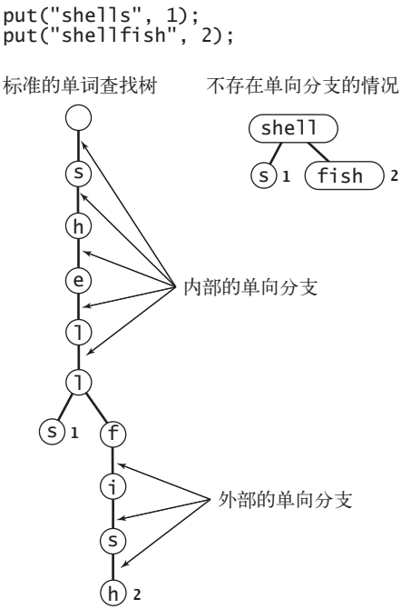
图 5.2.9 消除单词查找树中的单向分支
