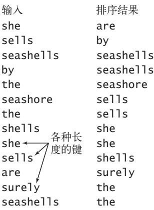
图 5.1.10 适于使用高位优先的字符串排序的典型情况
