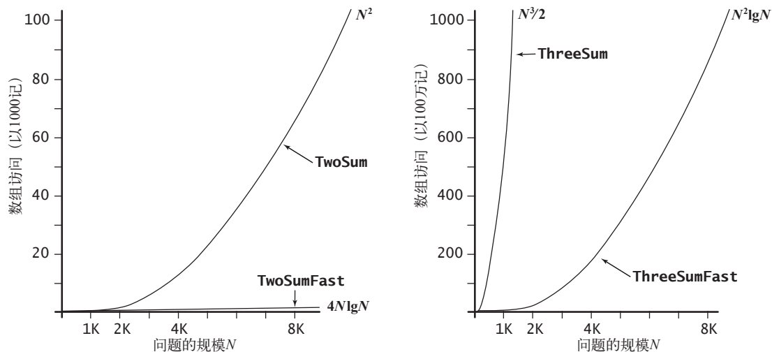
图 1.4.6 解决 2-sum 和 3-sum 问题的各种算法的成本
