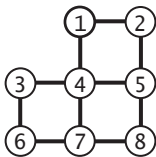
图 4.3.16
