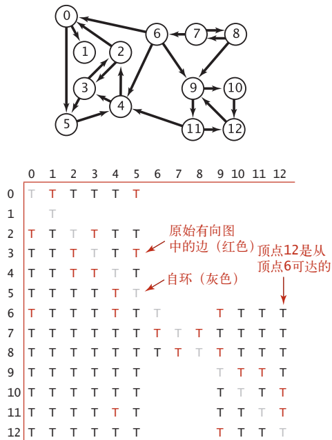
图 4.2.18 传递闭包
