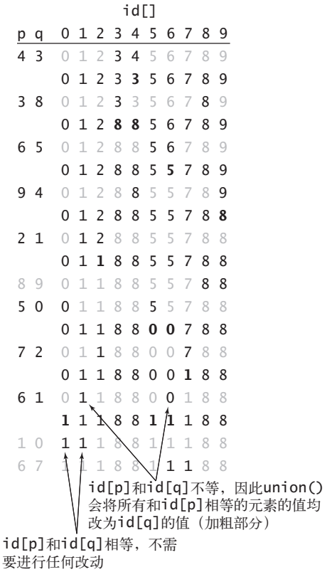
图 1.5.3 quick-find 的轨迹
