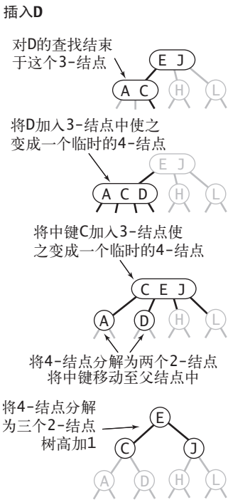
图 3.3.7 分解根结点
