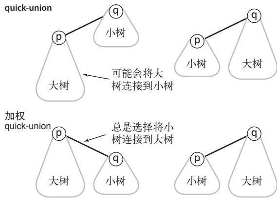
图 1.5.7 加权 quick-union
