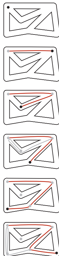
图 4.1.12 Tremaux 搜索
