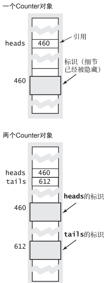
图 1.2.1 对象的表示
