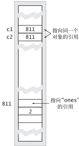
图 1.2.4 别名
