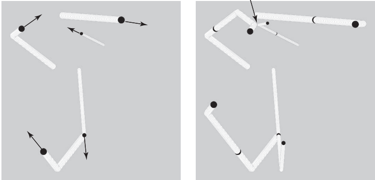
% java CollisonSystem 5
