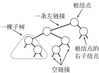
图 3.2.1 详解二叉树
