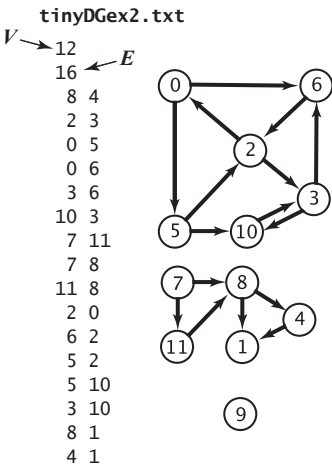
图 4.2.19
