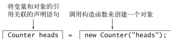
图 1.2.2 创建对象
