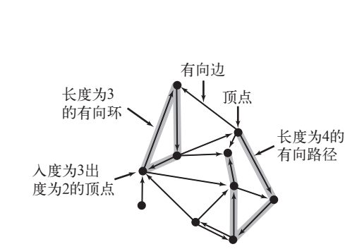
图 4.2.1 有向图详解
