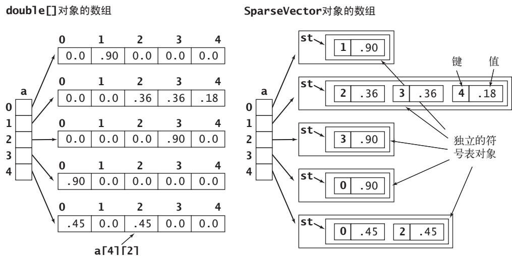
图 3.5.4 稀疏矩阵的表示
