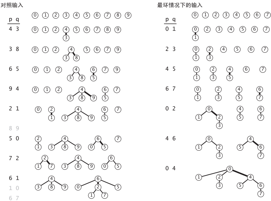
图 1.5.8 加权 quick-union 算法的轨迹（森林）
