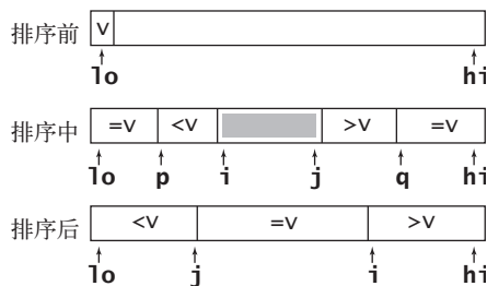
图 2.3.6 Bently-McIlroy 三向切分
