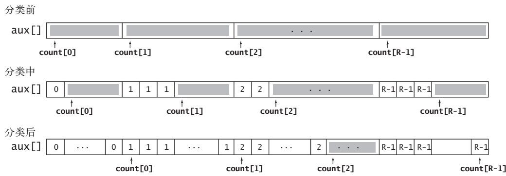
图 5.1.5 键索引计数法（分类阶段）
