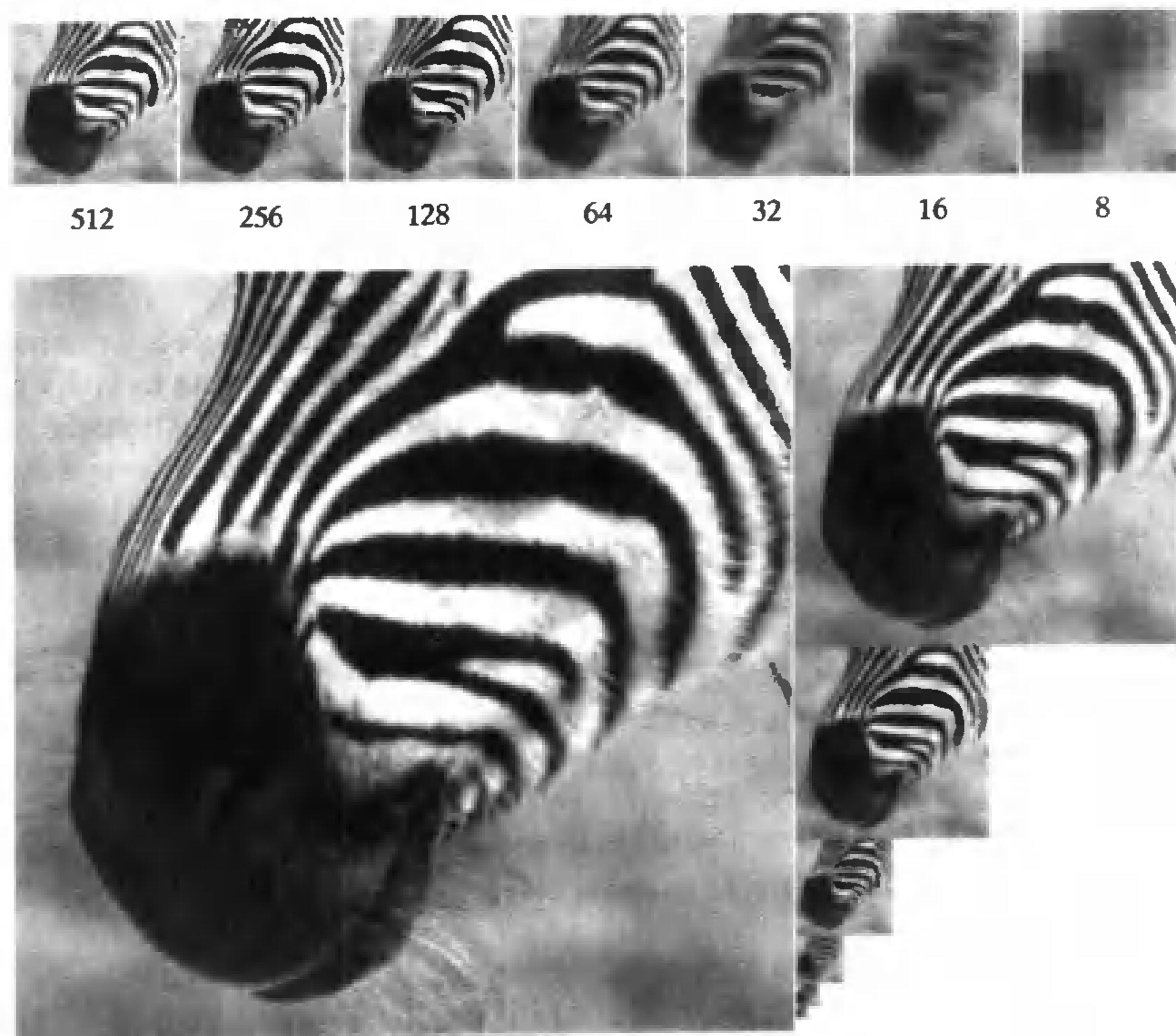
图 7.17 图像的高斯金字塔从 512 \times 512 到 8 \times 8 。上面一行中,把每张图以同样的尺寸显示(其中的一些像素尺寸较大),图的下面一部分是每张图的真实尺寸。注意到,如果将每张图与一个固定尺寸滤波器进行卷积,将获得截然不同的现象。最细粒度的图像中一个 8 \times 8 像素的块将包含一些绒毛;在粗一些的粒度中可能包含一个完整的斑纹,同时在最粗粒度中,包含动物的鼻子
