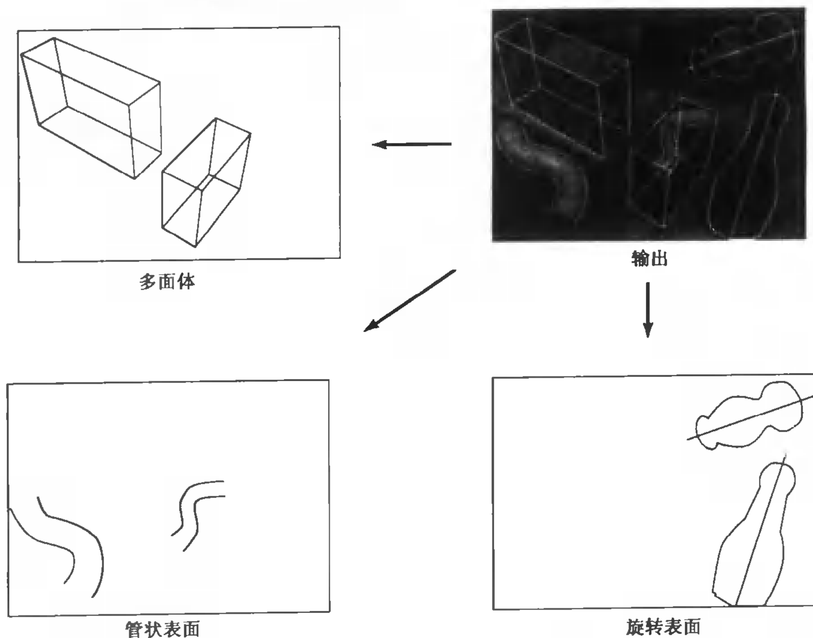
图 24.9 一个基于类别组合系统的例子:左图是一幅输入图像,它的边缘图表示在中图上。在右图上是表示不同类型的物体轮廓的曲线组。从图像中检测出的边缘往往有断点、遮挡点等。但它们可在对具体类型物体的处理过程中加以修补(例如,多面体组合器修复线段上的问题,旋转表面组合器使用镜像对称来修补镜像对称曲线对中丢失的信息等)。因为每类使用略有不同的组合器,轮廓的分类在过程的结局中确定,但是分类只取决于物体的类型,而不是具体的哪一个物体,更加详细的例子显示在图24.10
