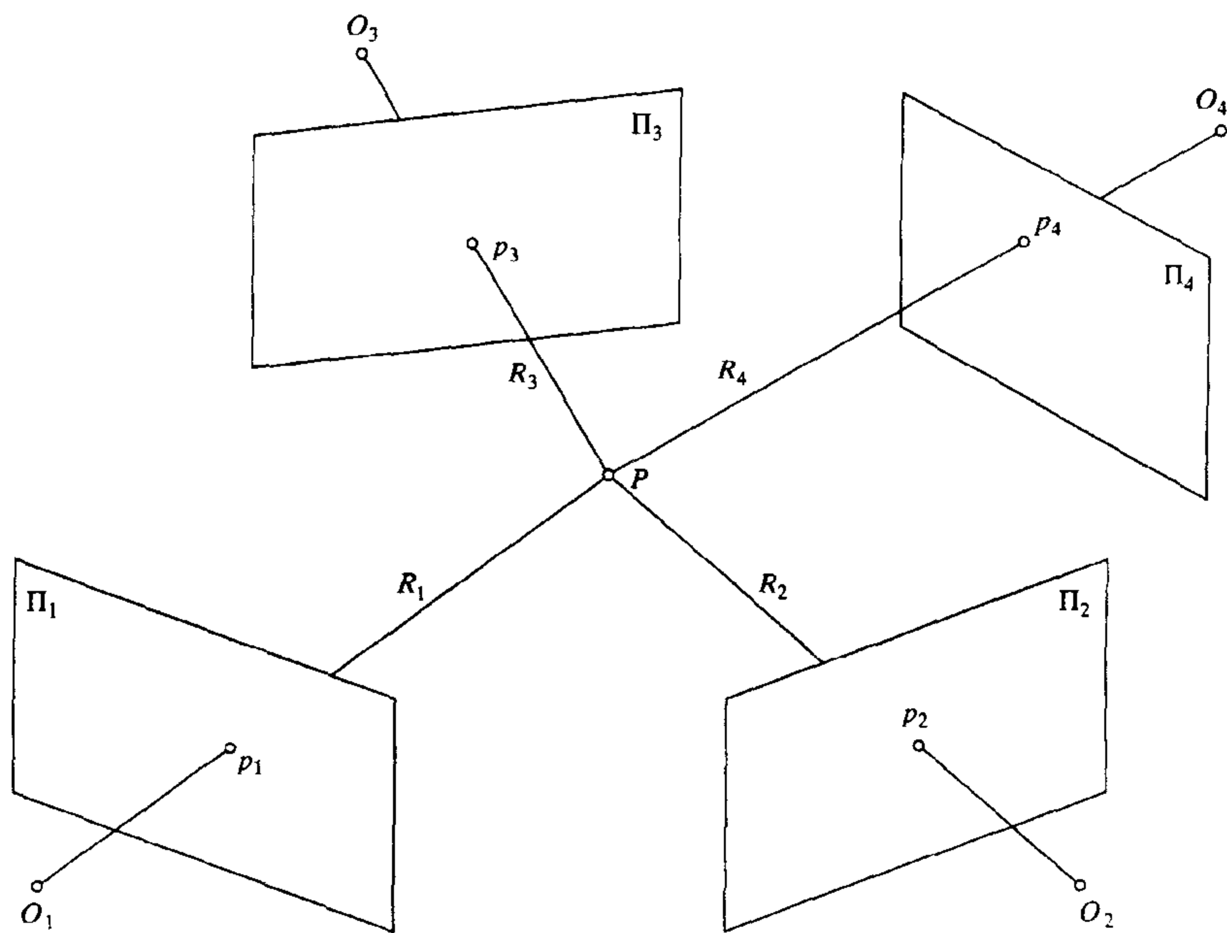
图 10.8 点 P 在 4 个视图中的像点是这 4 个像点相应射线的交点。点 P 的 4 个像点 p_1, p_2, p_3 和 p_4 确定了该点是对应的 4 条射线 R_i ( i = 1, 2, 3, 4 ) 的交点。
