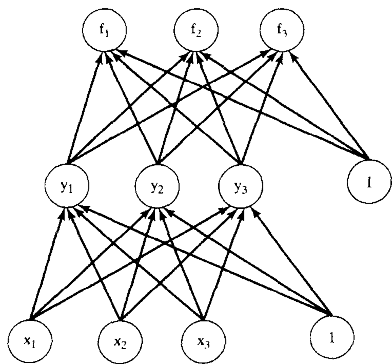
图 22.12 神经元网络通常可以用上述形式的图来描述。图中的每个圆圈表示一个神经元变量,通常圆圈中会有一个标号。网络的层次结构可以从图中表现出来,如上图所示的是一个两层神经元网络,不同层用的变量符号不同,箭头表示在仿射变换中连接两个神经元之间的非零系数。由于上图中任意两个结点都有箭头连接,因此上图所示的网络是全连接的。请注意,图中可能会出现跨层的箭头
