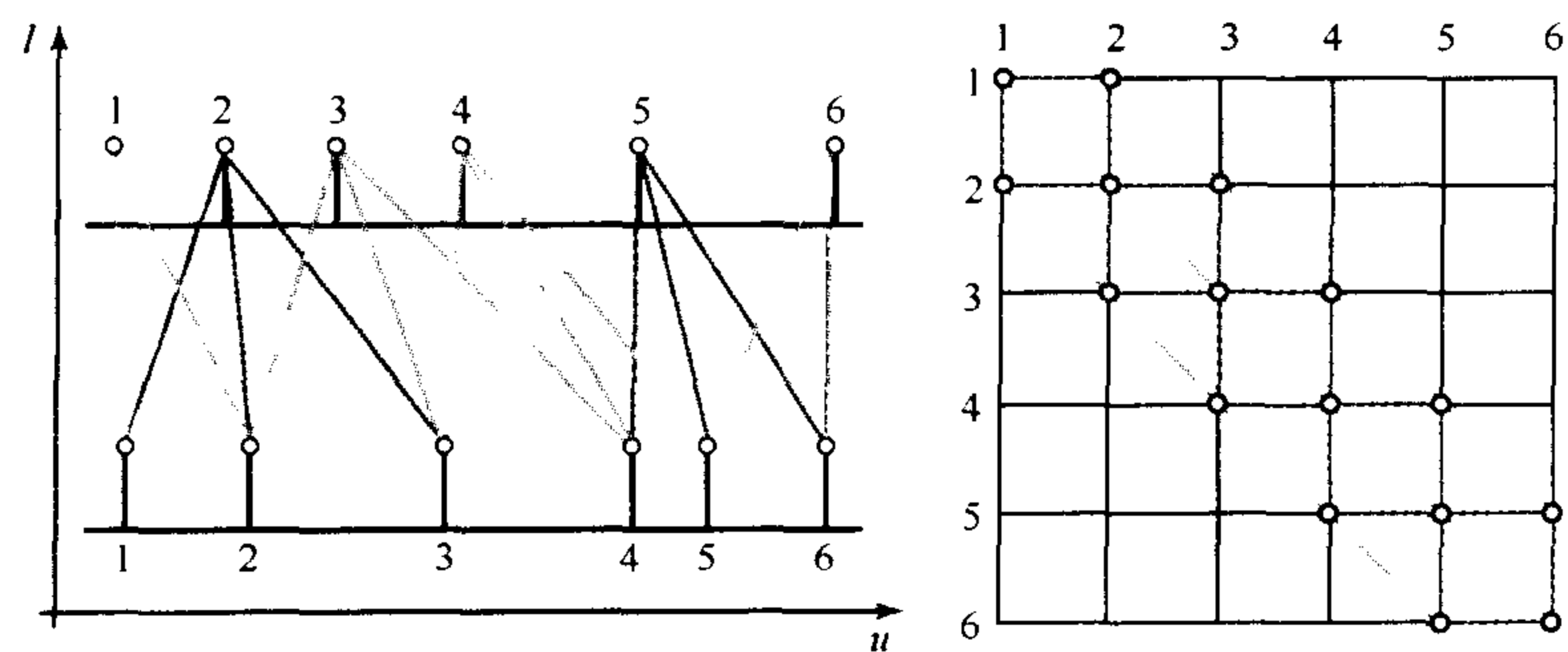
图 11.7 一个协作方式工作的立体分析方法：Marr-Poggio 算法(1976)。左图展示了两幅图像沿着同一扫描线的灰度轮廓。每个钉子状的图示代表一个黑点。连接两个黑点的线段意味着在一定的最大视差范围可能的匹配。这些匹配在右图中也有显示，右图是这些节点形成的一个图。垂直和水平弧连接的节点表示了左图或右图中同一个点。对角线弧连接了具有相似视差的节点
