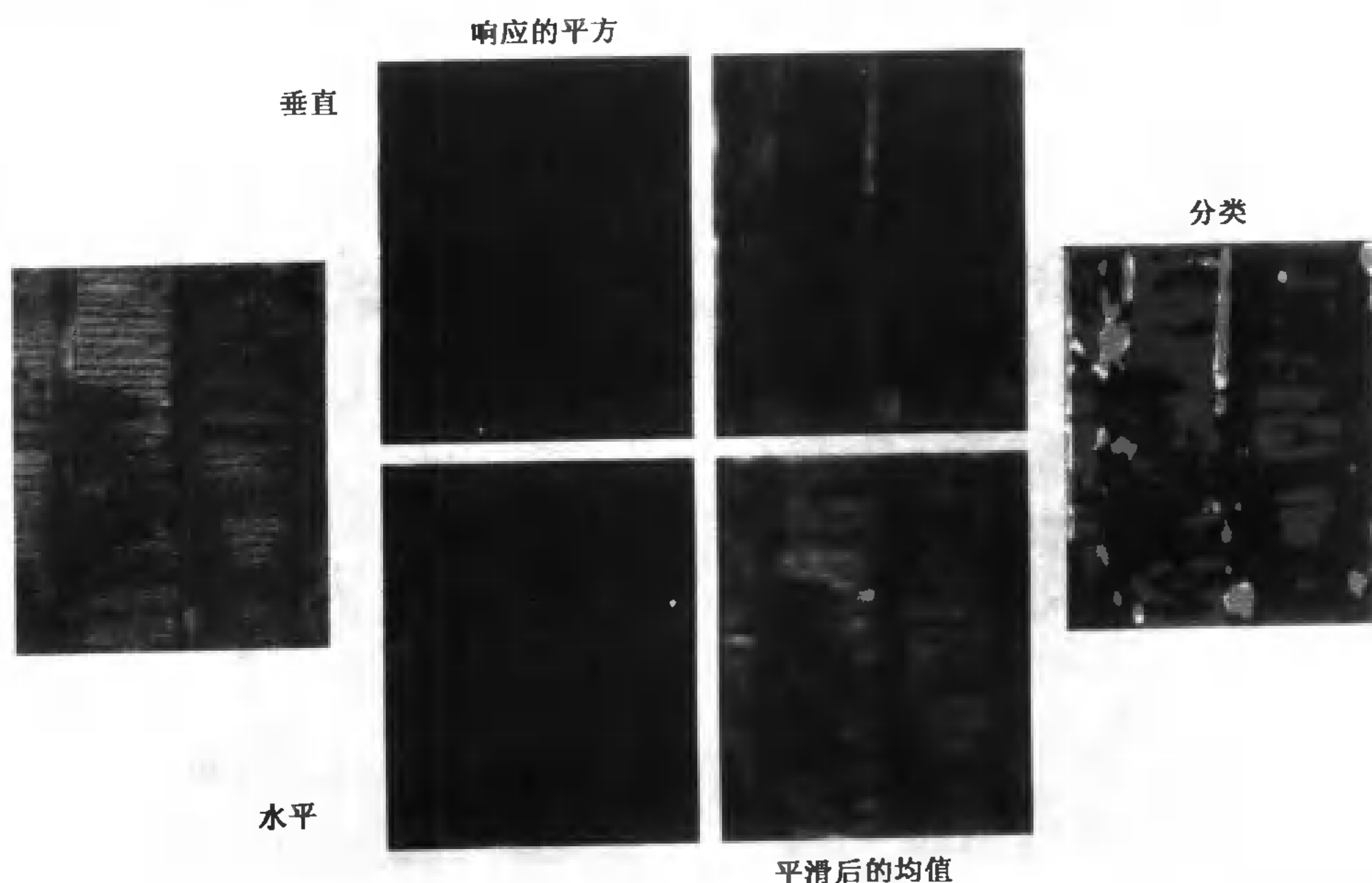
图 9.6 一个根据滤波器输出结果假定的描述。我们明显地减少了滤波器的数量(有两个不同的滤波器,一个垂直,一个水平)。左边的图像是输入,注意可以将它的各部分可靠地描述为垂直的,或是水平的,或是模糊的。中间左边那一列的图像是平方后的滤波输出结果(平方是用来使从黑色到白色的转变和从白色到黑色的转变相同)。这些值用同样的线性尺寸来显示,来使从黑色到白色的转变和从白色到黑色的转变相同)。这种平均响应使垂直的条纹在垂直的图像中更加明显,水平的条纹在水平图像中更加明显。最后,阈值化两幅图像,然后合并它们得到右边的图像。(黑色的值既不是垂直也不是水平,深灰度的值是水平,浅灰度的值是垂直,白色的值是水平且垂直)
