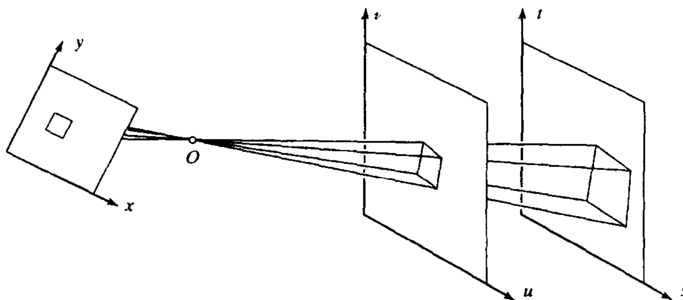
图 26.15 从图像获取一个光线极板,从光线极板合成新图像,可用 (x, y) 图像平面和定义光线极板的 (u, v) 和 (s, t) 平面间的透视变换建模
