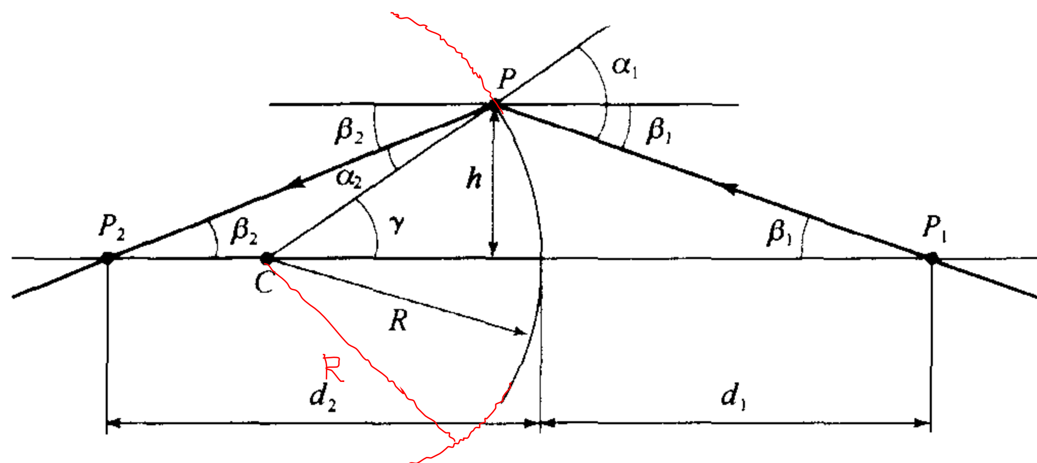
图 1.8 近轴折射:一条穿过 P_1 的光线在点 P 与一个圆形界面相交,并发生折射。折射光穿过点 P_2 ,界面中心在光轴上的点 C ,半径为 R 。假设角度 \alpha_1, \beta_1, \alpha_2 与 \beta_2 都很小
